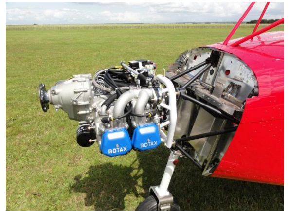
Mise en place du moteur sur le bâti
